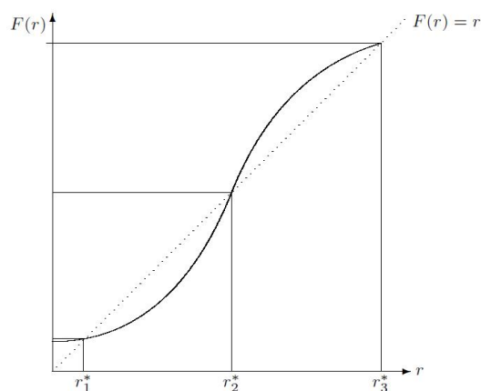
ABBILDUNG 12.1: GLEICHGEWICHTE IM SCHWELLENWERTMODELL
